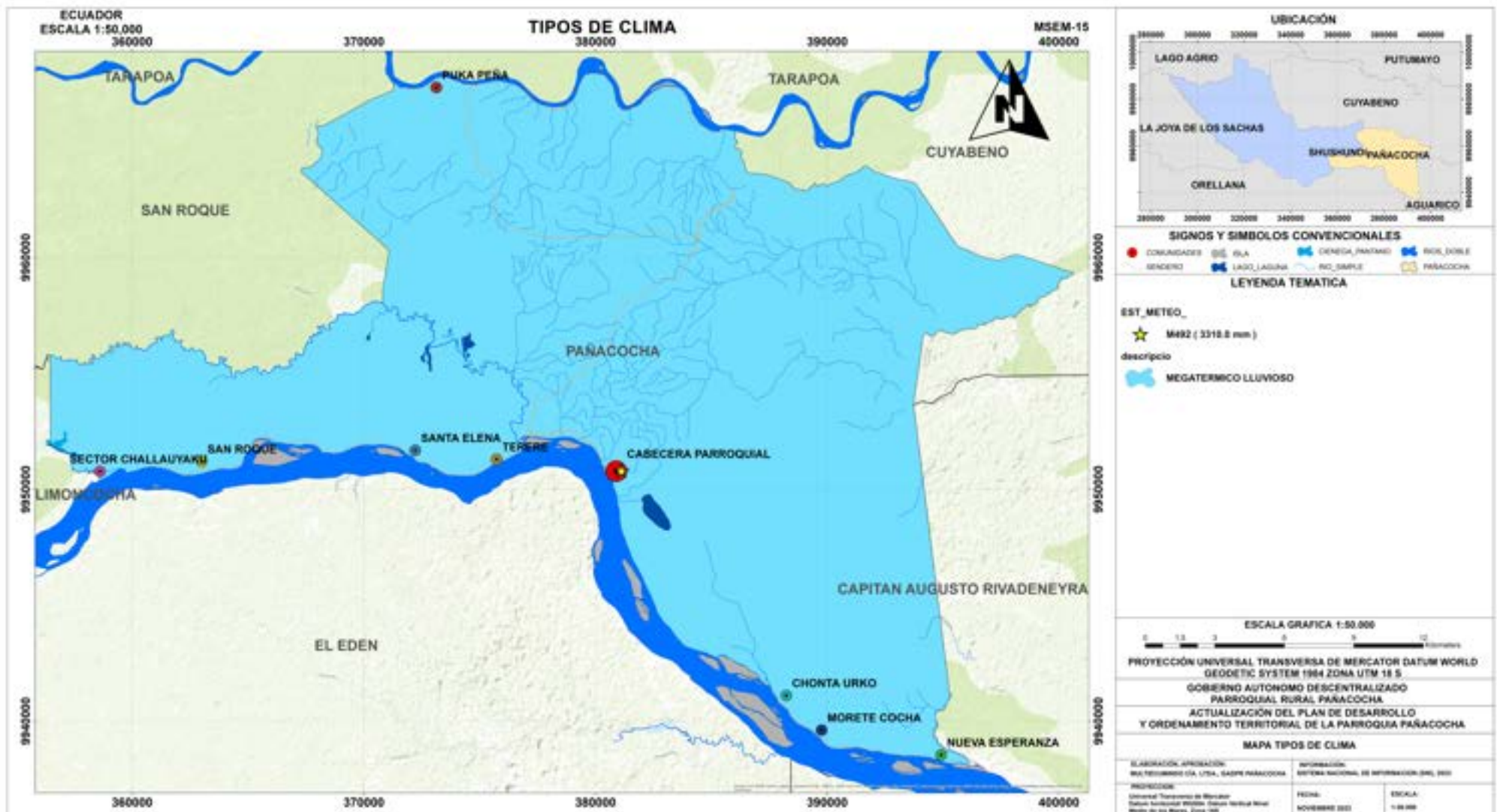
Mapa N° 15. Tipo de clima.
