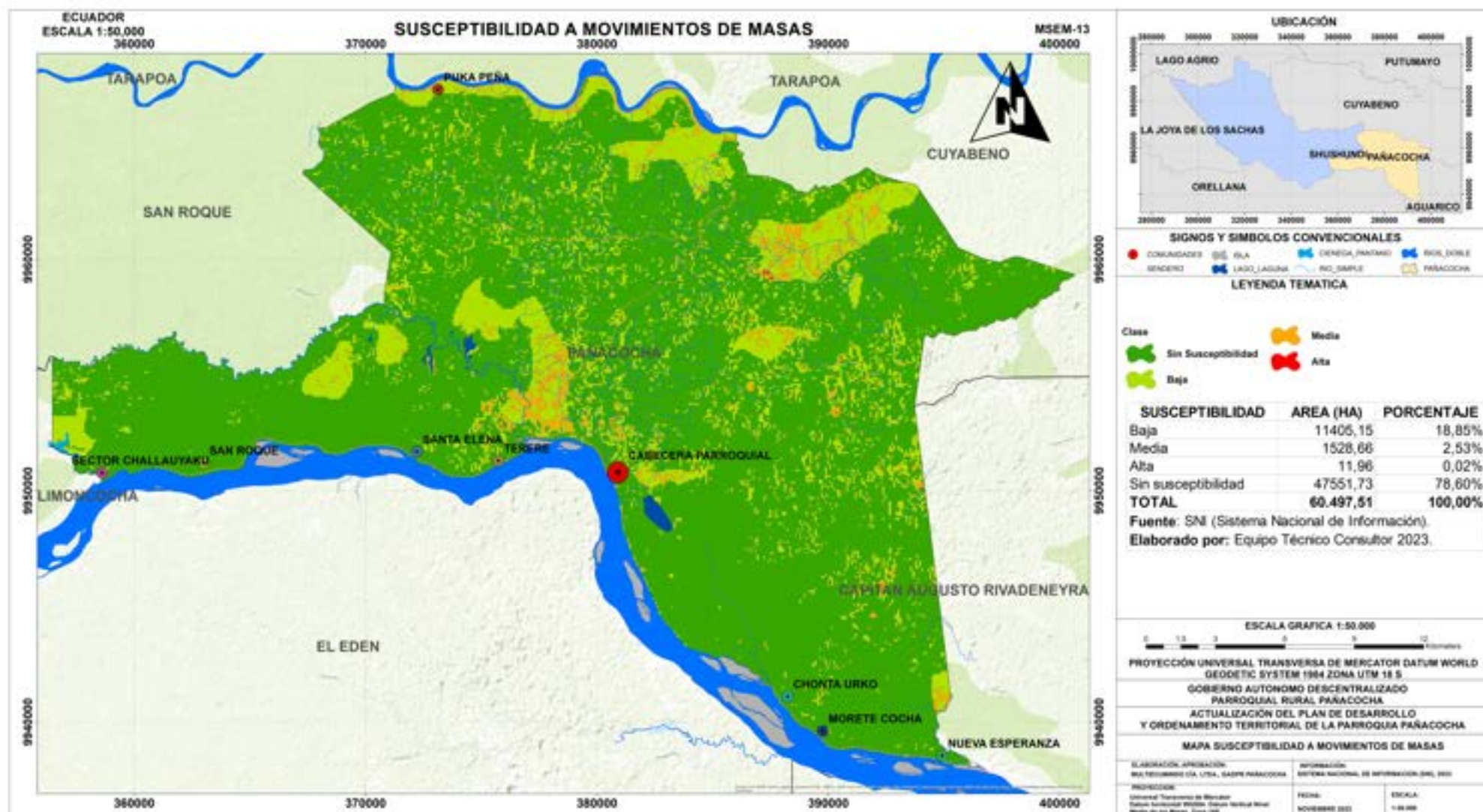
Mapa N° 13. Susceptibilidad a movimientos en masa
