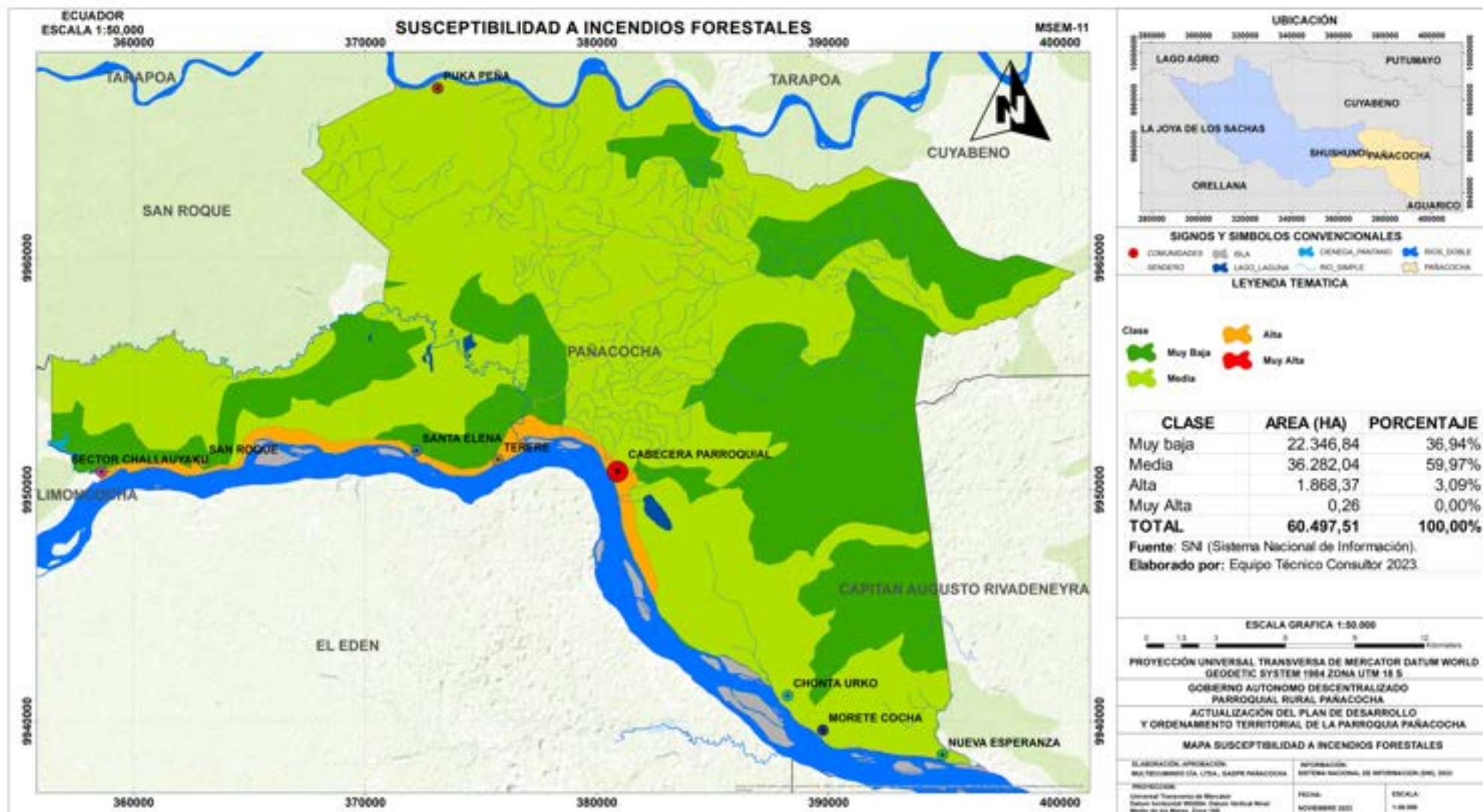
Mapa N° 11. Susceptibilidad a incendios forestales
